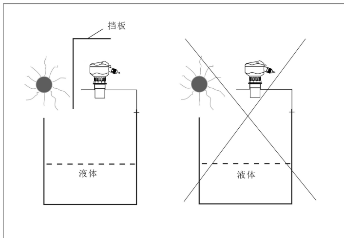
温度变化大--加遮阳板或者仪表箱
