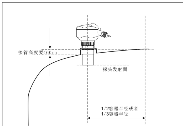
安装在螺纹接管上--拱形罐顶
