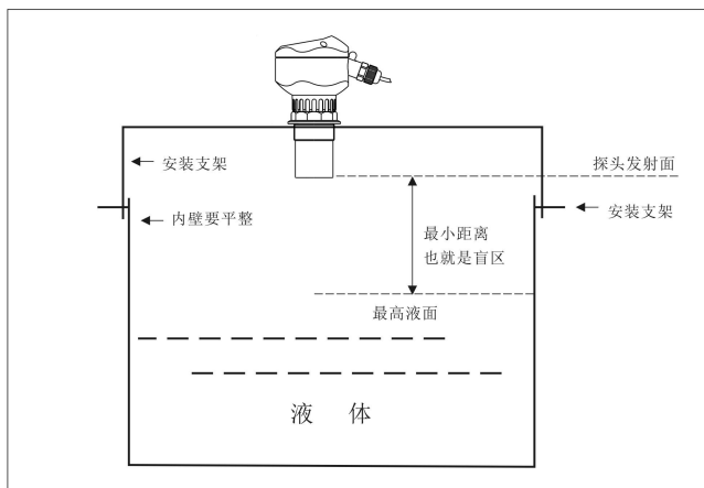
开口容器上--顶部居中支架安装
