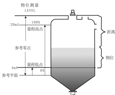
附图 1.2 物位测量示意图
