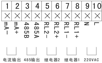
四线制 220VAC 供电接线图
