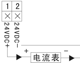
一体式防爆型二线制跟电流表连接
