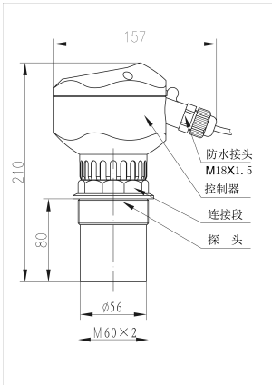
螺纹 M60×2 传感器
