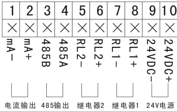
四线制 24VDC 供电接线图
