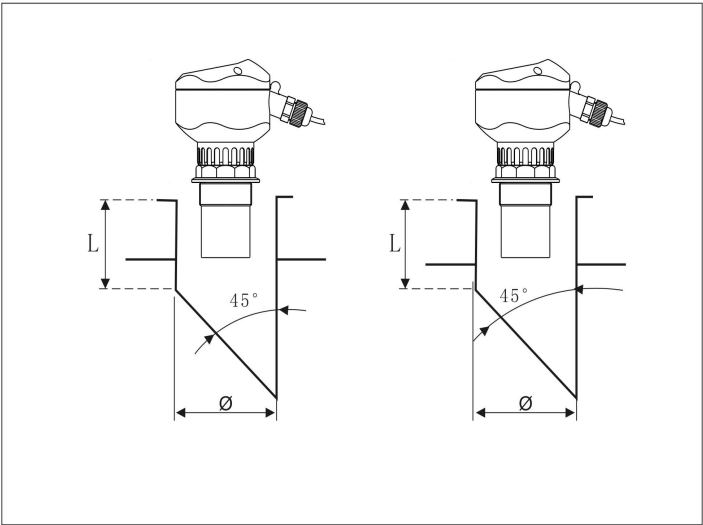
不浸泡在介质中的延长接管
