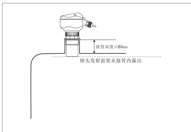
探头安装在螺纹接管上
