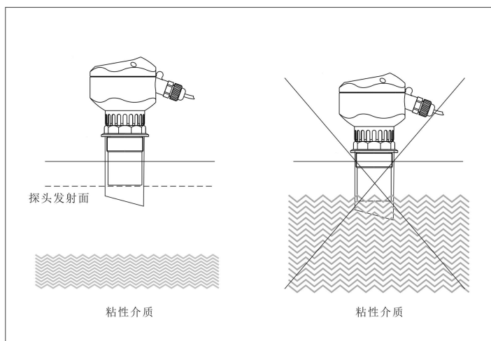
接管不能浸泡在粘附性介质里
