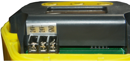
二线制电气连接图
