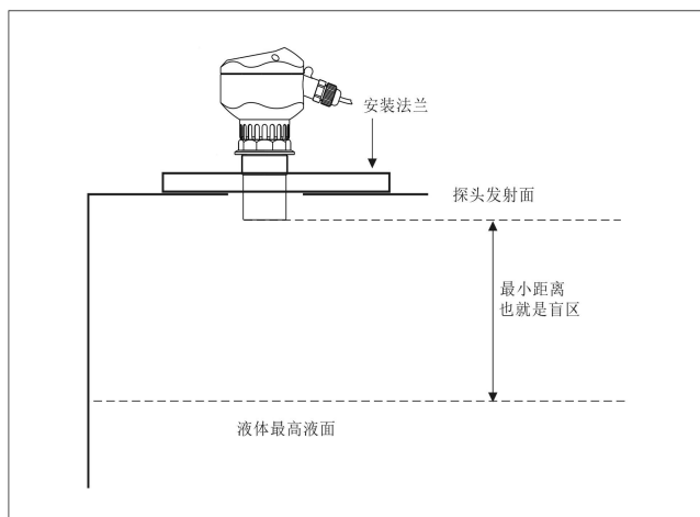
法兰型（锁紧法兰），安装在平顶罐上
