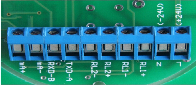
一体式防爆型四线制电气连接图
