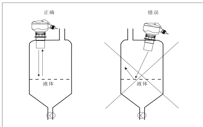
传感器探头应垂直于介质表面
