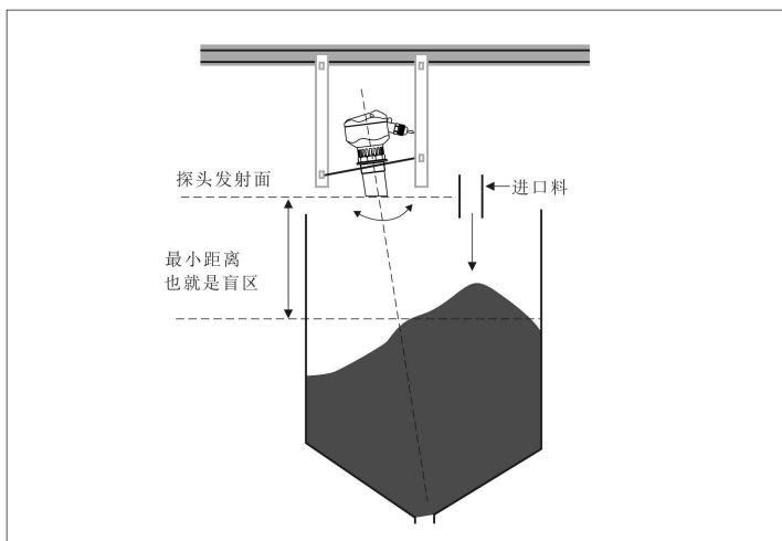
一体式传感器—龙门框安装
