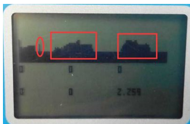
图 8 变频器干扰的回波图形
