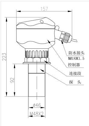
螺纹 M48×2 传感器
