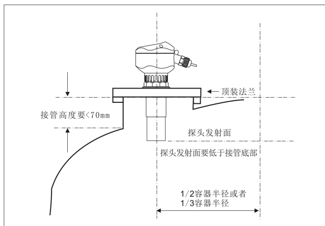
安装在法兰上--拱形罐顶
