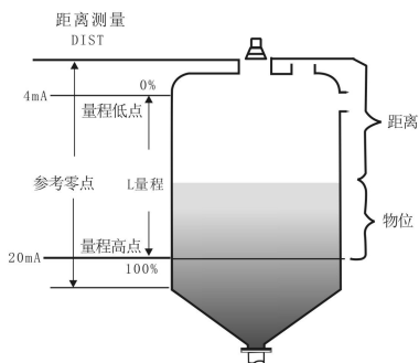
附图 1.1 距离测量示意图
