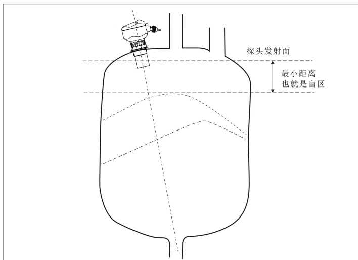
一体式传感器—螺纹接管安装
