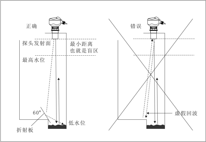
水池底部有障碍物—用挡板折射走
