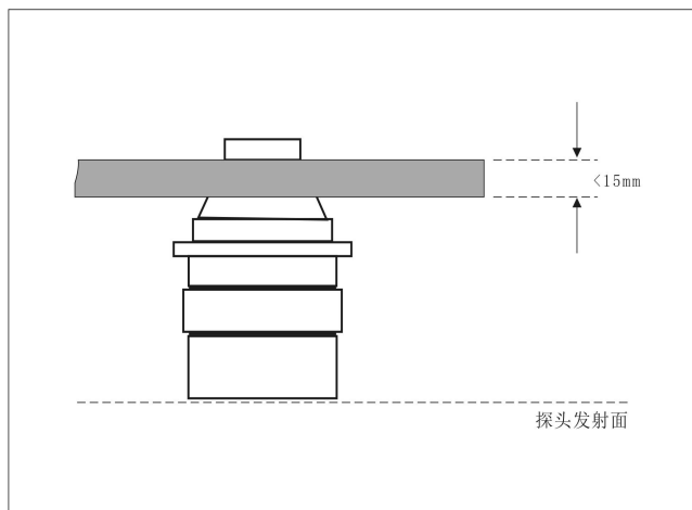
分体式探头顶部吊装螺纹连接
