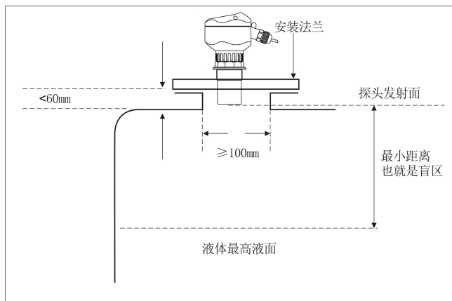
法兰安装，安装在很短的接管内
