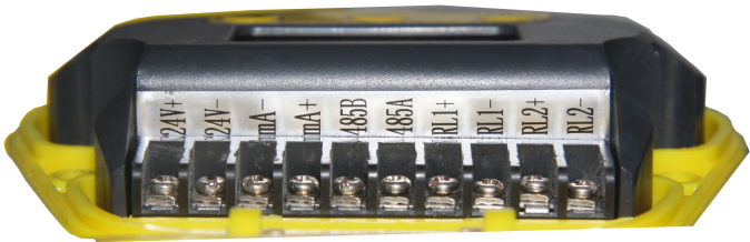
一体式增强型四线制电气连接图
