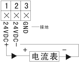
二线制接电流表示意图
