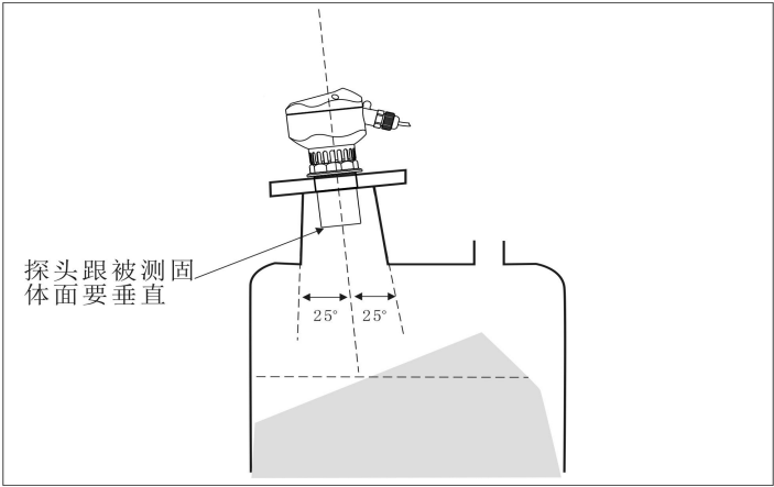
测量固体介质的延长接管
