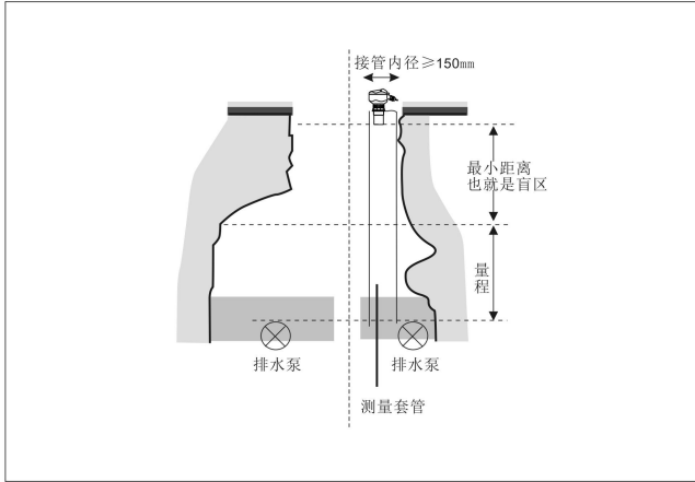
接管和测量套管用于排水井测量
