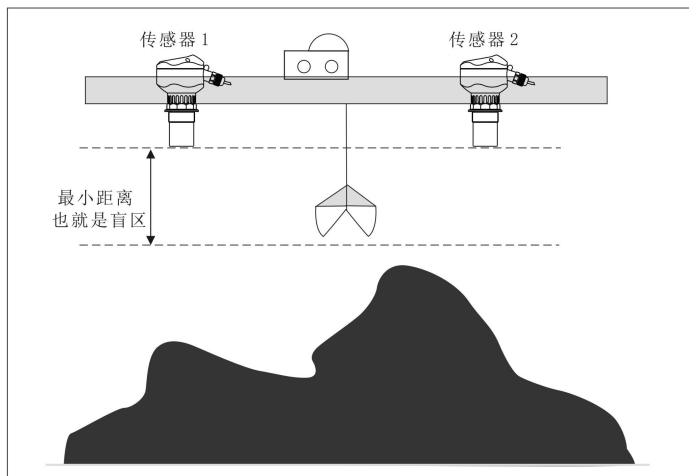
露天料堆测量—起重架上安装
