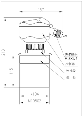
螺纹 M108×2 传感器
