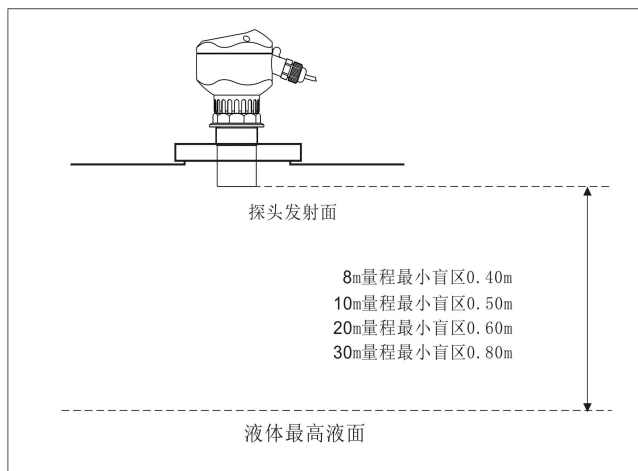
法兰型安装在无接管平项罐上
