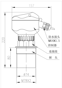
螺纹 M78×2 传感器
