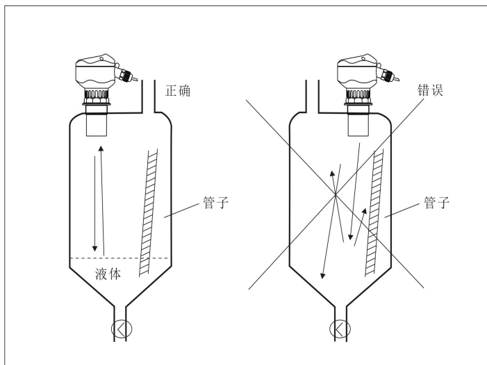
容器内的障碍物--管子
